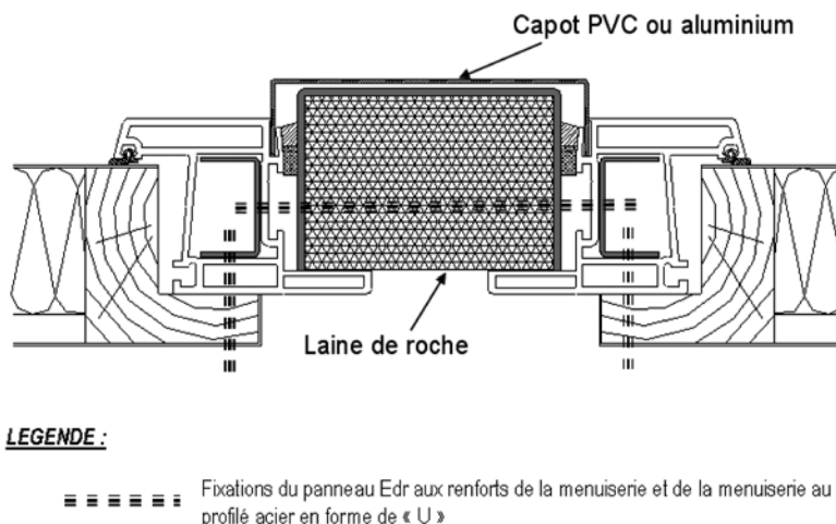
Figure 16 : jonction entre fenêtres ou ensembles menuisés
