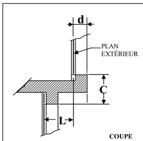
Figure A2 : règle de calcul du D, d < 0,15 m
