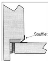
Figure 9 : exemple de soufflet au-dessus du plancher
