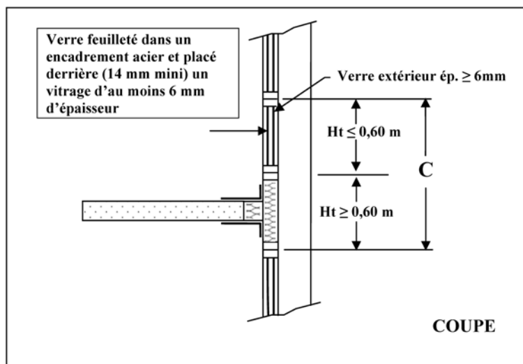
Figure 2c : cas particulier de complément de C en verre feuilleté
