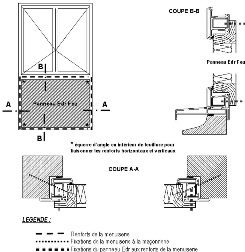
Figure 14 : panneau de façade à ossature en PVC posé au plus au nu extérieur de la façade (nu extérieur de la fenêtre aligné au mieux ou en retrait de moins de 10 cm avec le nu extérieur de la façade)
