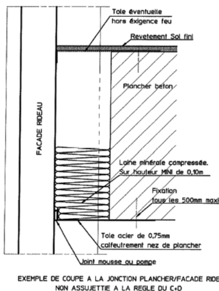
Figure 23 : exemple de jonction façade/plancher lorsque le C + D n'est pas appliqué
