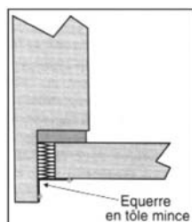
Figure 11 : autre exemple de dispositif devant le nez de plancher
