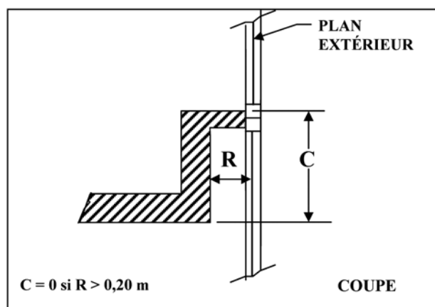
Figure A4 : allège en retrait d'une façade entièrement vitrée
