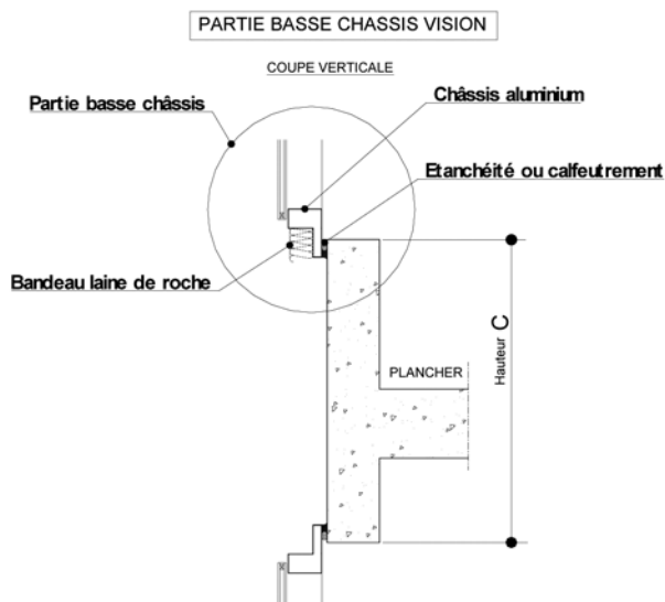
Figure 7 : étanchéité en périphérie des châssis vision
