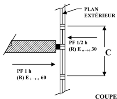
Figure 2b : résistance au feu des éléments participant au C
