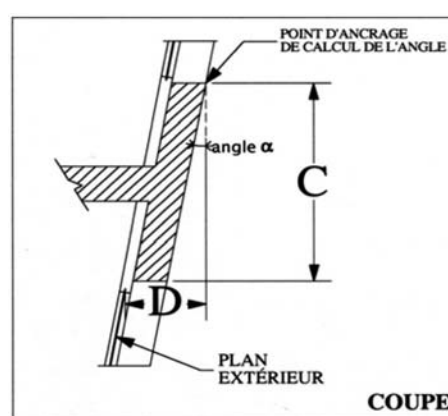
Figure A6 : façade inclinée vers l'extérieur
