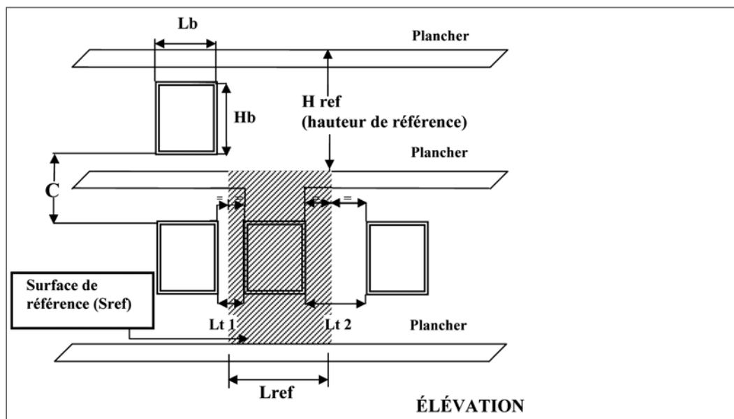
Figure 24 : définition de la surface de référence Sref
