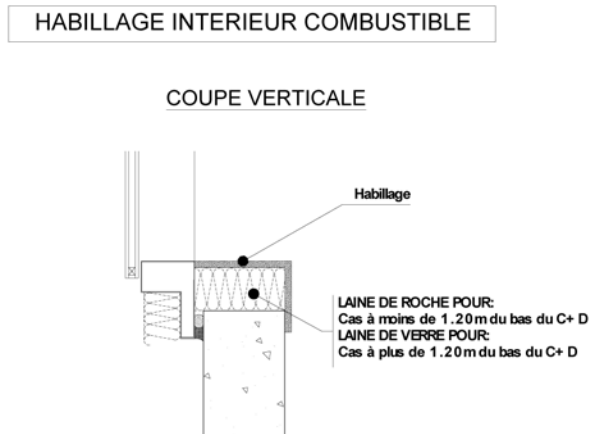
Figure 8 : protection des habillages intérieurs combustibles
