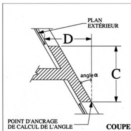
Figure A5 : façade inclinée vers l'intérieur
