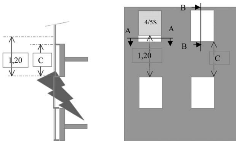
Figure 6 : principe de façade semi-rideau
